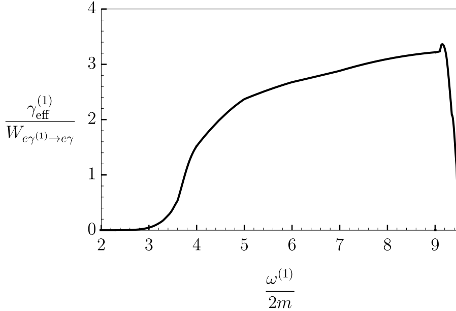
Рис. 12: Отношение коэффициента затухания фотона \gamma_{eff}^{(1)} к коэффициенту поглощения фотона в процессе e\gamma^{(1)} \rightarrow e\gamma при B = 200B_e и T = 1 МэВ
