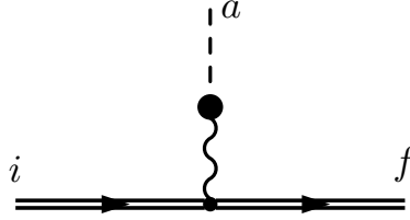
Рис. 14: Диаграммы Фейнмана для процесса общего вида i \rightarrow f + a . Двойные линии означают, что влияние внешнего поля на начальное и конечное состояния учтено точно.
